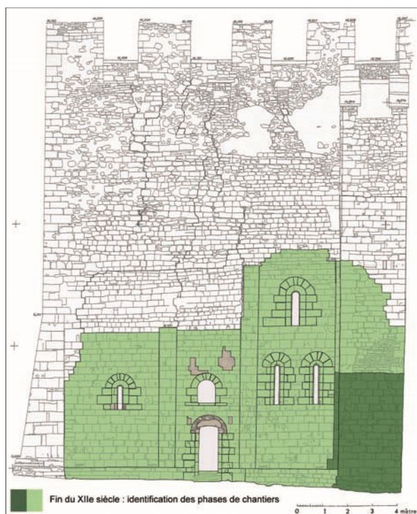
FIG. 12. ÉLEVATION SUD. Analyse des procédés constructifs et phasage.
