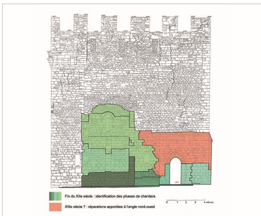
FIG. 8. ÉLÉVATION NORD. Analyse des procédés constructifs et phasage. A. Charrier, d'après les relevés photogrammétriques de 1972, Médiathèque du patrimoine, cote 1996/081/0032 et 1996/091/.
